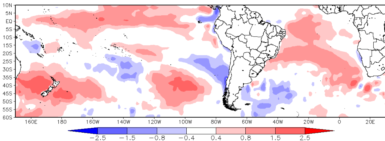
Figura 3. Anomalia Mensal de TSM calculada para março/2019 (UFPEI-CPPMet). Fonte dos dados: NOAA-CDC.
