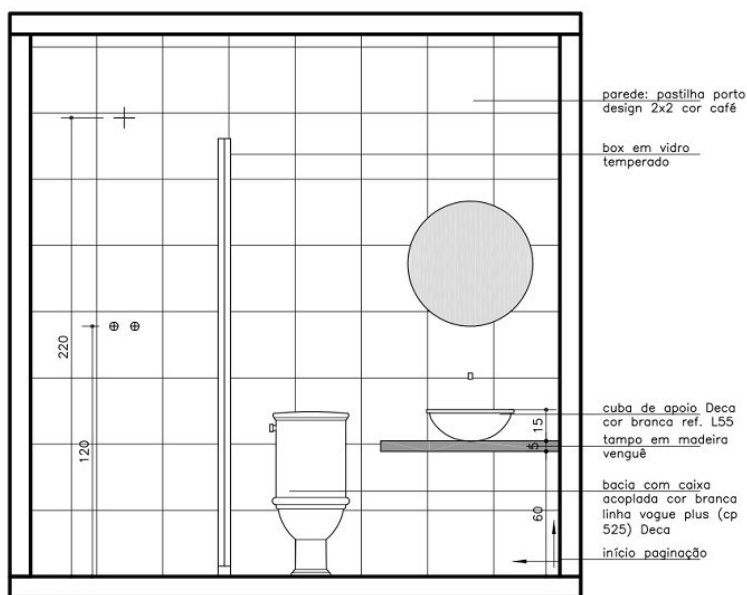
Vista Sanitário
