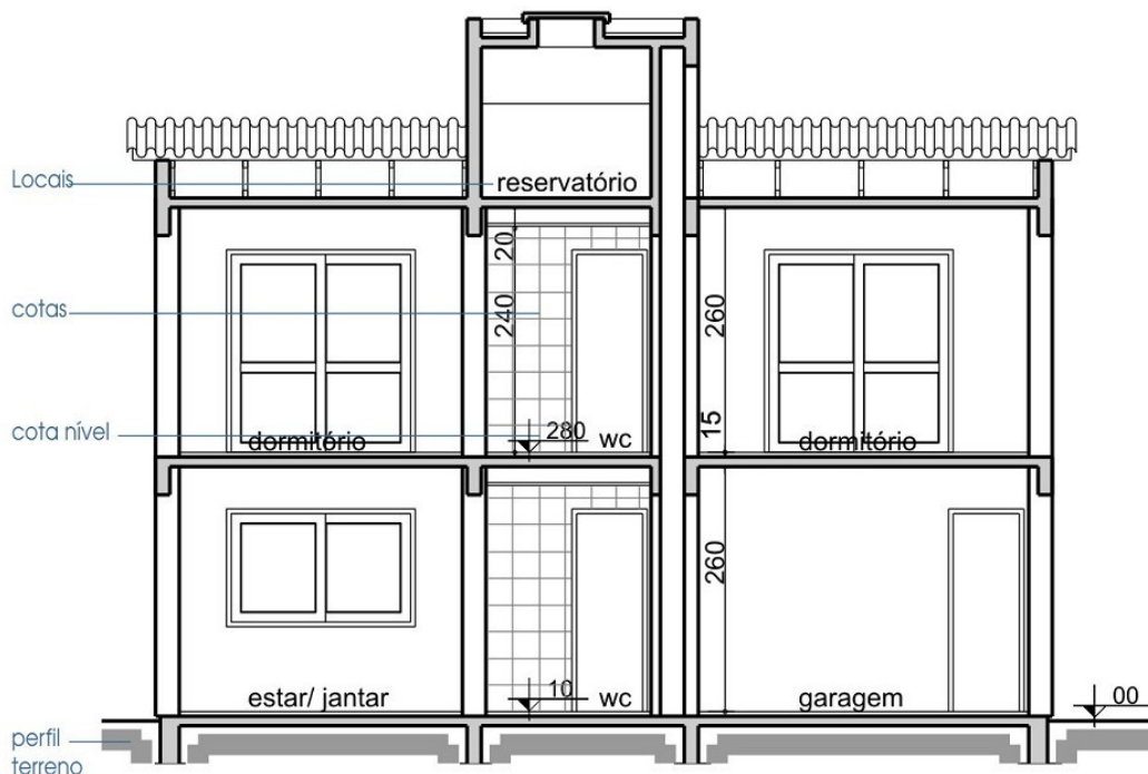
Corte A-A
