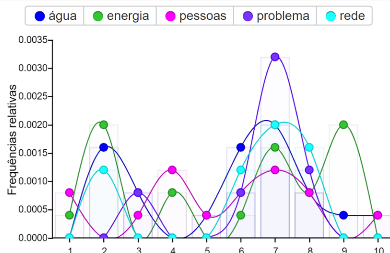
Figura 28. Fonte: https://voyant-tools.org/
