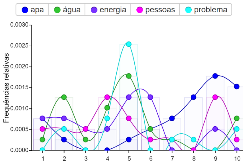
Figura 37. Fonte: https://voyant-tools.org/
