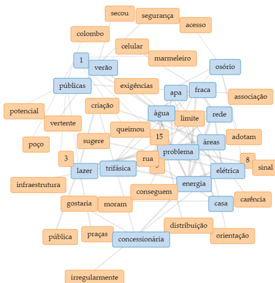
Figura 36. Fonte: https://voyant-tools.org/
