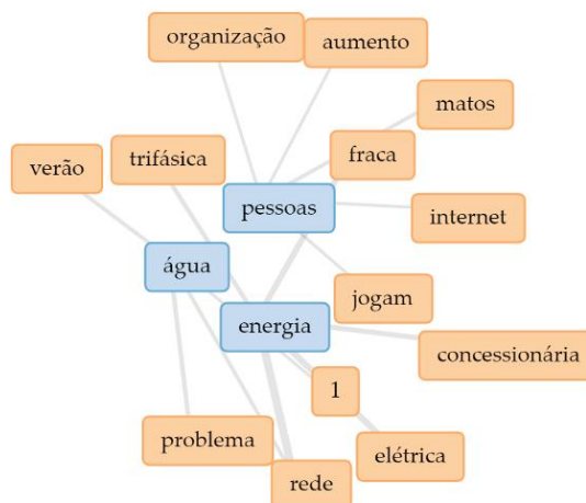
Figura 27. Fonte: https://voyant-tools.org/
