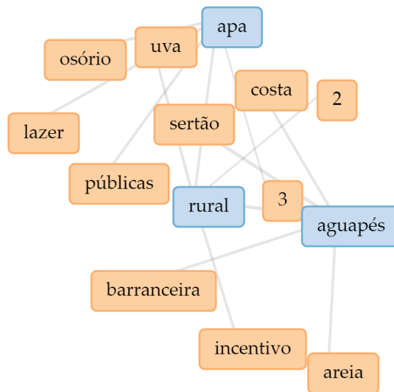
Figura 33. Fonte: https://voyant-tools.org/
