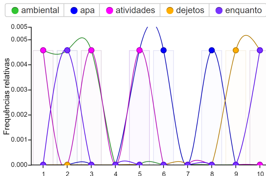
Figura 31. Fonte: https://voyant-tools.org/
